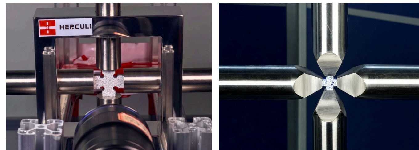
双轴试验
