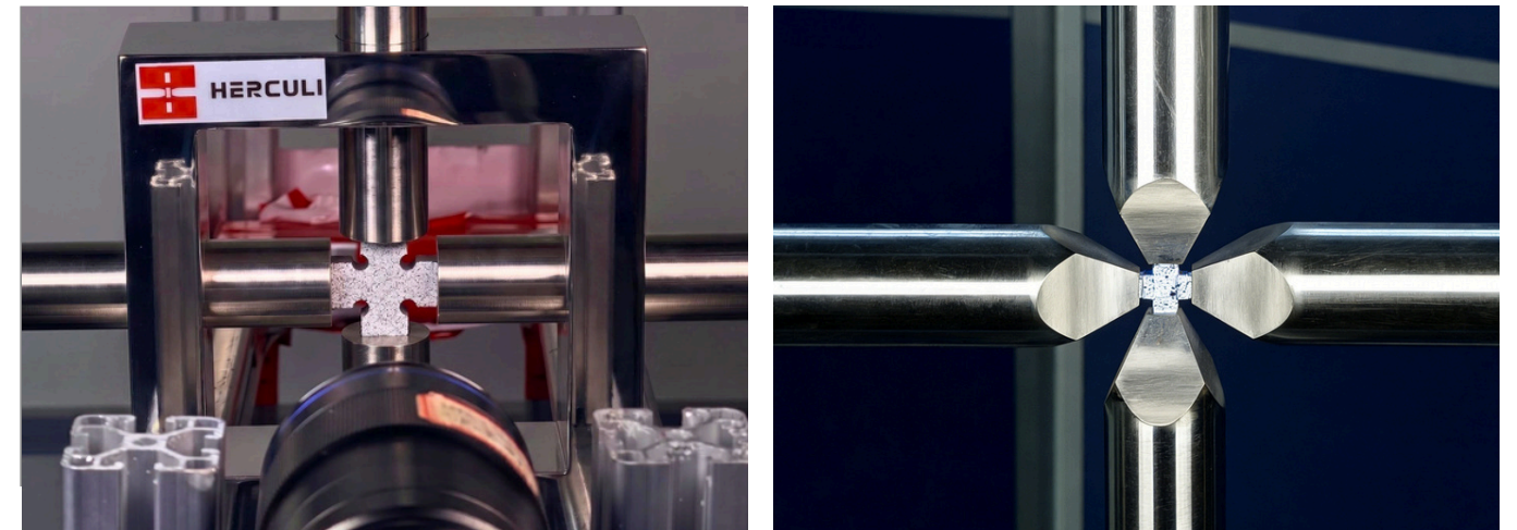
双轴试验
